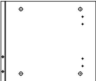
4. 409x348x16 mm
