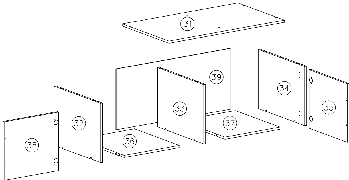
WYMIARY ELEMENTÓW PART GUIDE MASSE DER BAUTEILE
