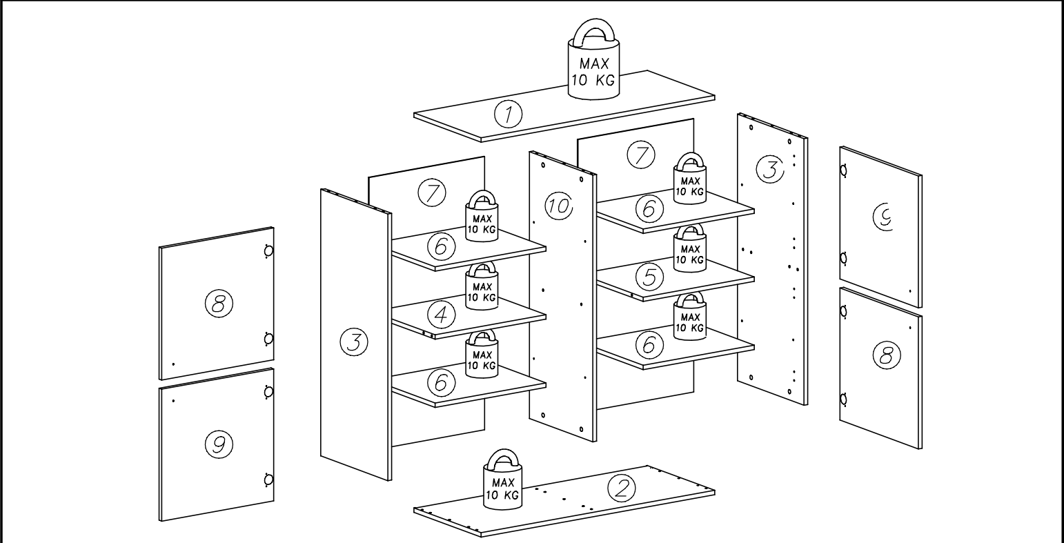
WYMIARY ELEMENTÓW PART GUIDE MASSE DER BAUTEILE
